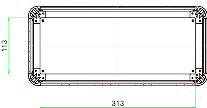
C-C ( 1 : 4.5 )
