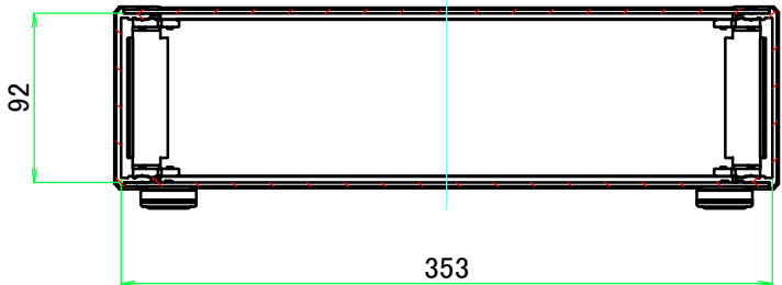
A-A ( 1 : 4.5 )
